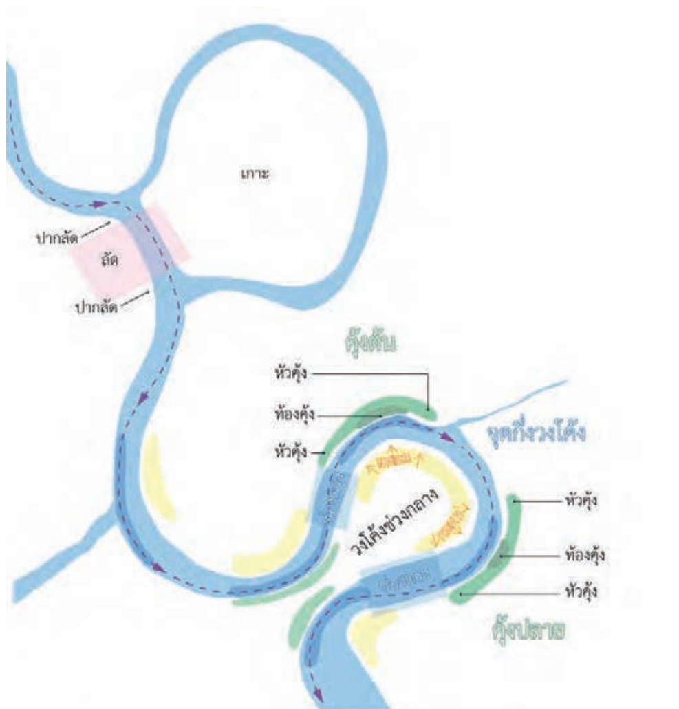
ภาพจำลองภูมิลักษณะของสัณฐานของลำน้ำโค้งตวัด
